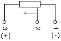
Potansiyometre bağlantısı ( Gerilim Bölücü )
