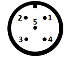
M12 / 5 Pin erkek soket (kablo takılan soketin karşıdan görünümü)
